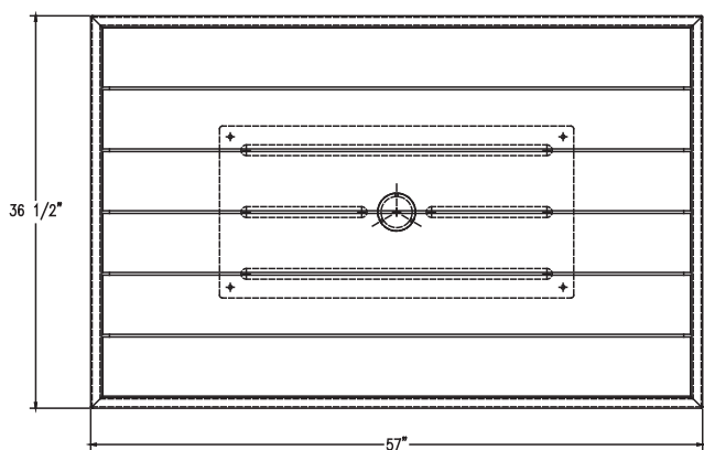
TOP VIEW 1033 ADA
