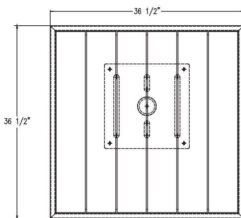
TOP VIEW 1049 ADA
