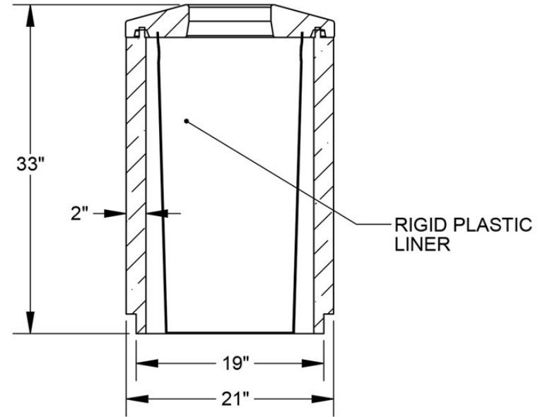
SECTION A-A SCALE 1 : 14
