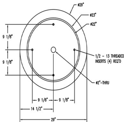
3 BOTTOM VIEW Scale: 1/8" = 1"
